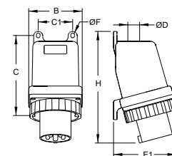
Ölçüler (mm)
